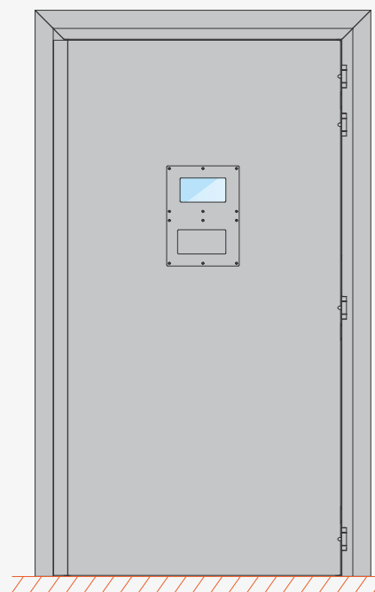
Aanzicht scharnierzijde met doorgeefluik
