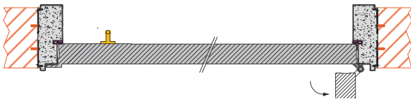
Aanzicht tunnelplaatsing
