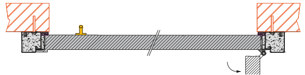
Aanzicht opbouwplaatsing
